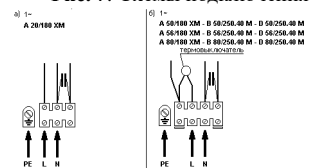
Рис. 7: Схемы подключения электропитания
