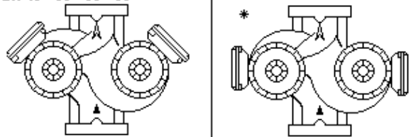
Рис. 3. Неправильная установка насосов.
